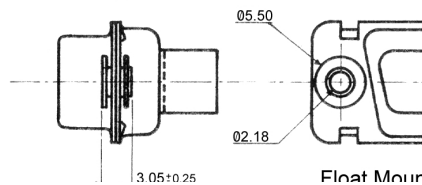
Montage Flottant
