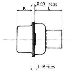
Montage Flottant
